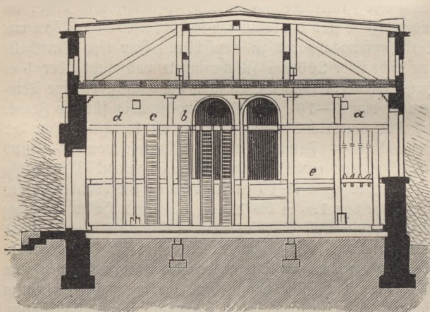
Turmhalle: Durchschnitt.
